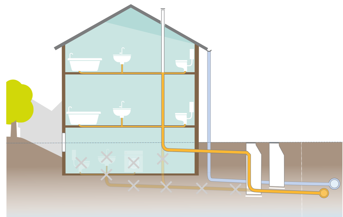
Abbildung 19: Rückbau von Entwässerungsgegenständen im Keller
