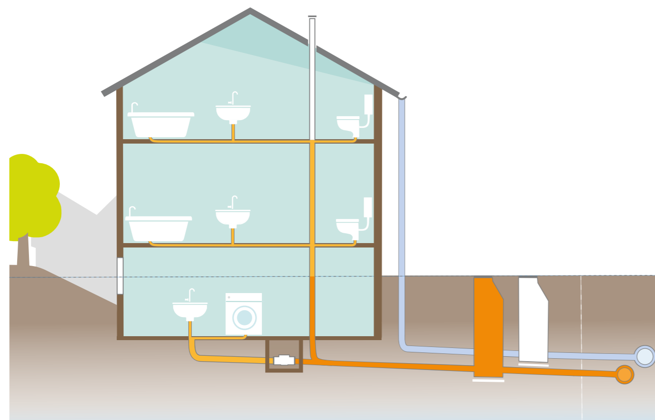
Abbildung 17: Rückstauverschluss
