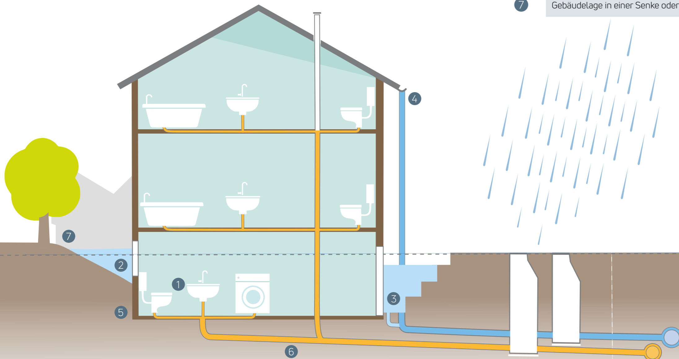
Abbildung 12: Wassereintrittsmöglichkeiten am Haus
