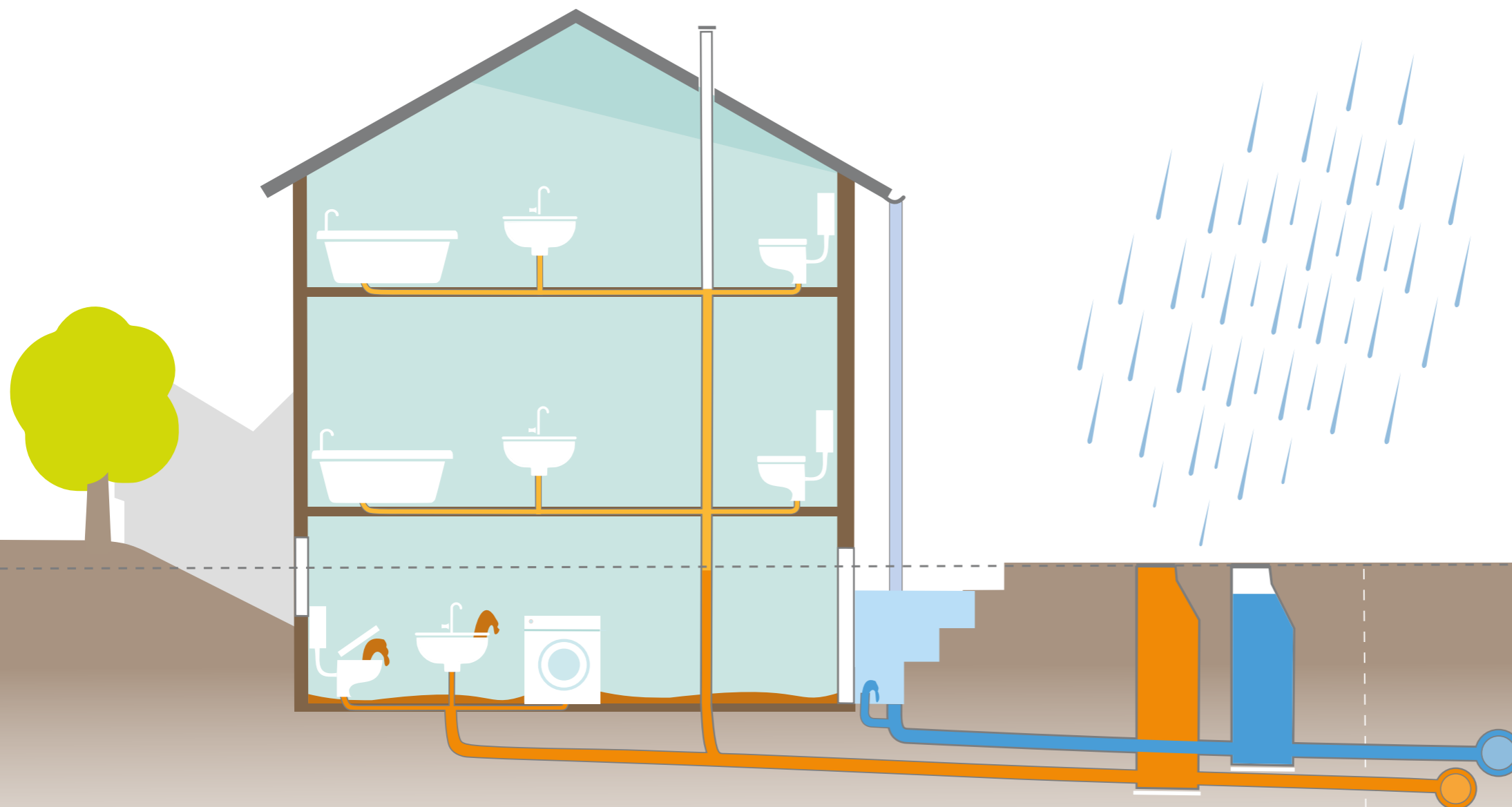
Abbildung 13: Überflutungsrisiko bei fehlendem Rückstauschutz
