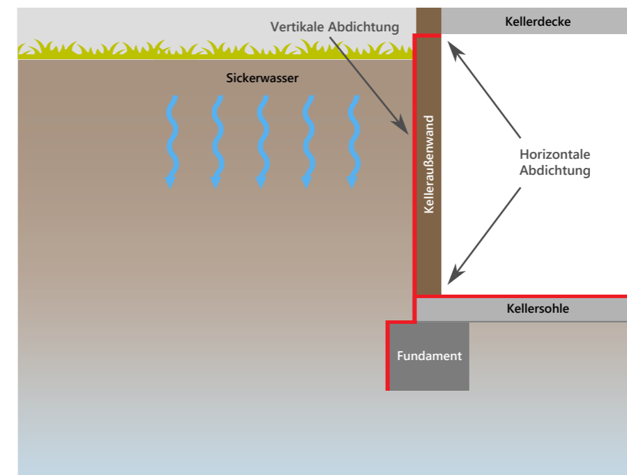
Abbildung 29: Abdichtung bei Auftreten von Bodenfeuchte
