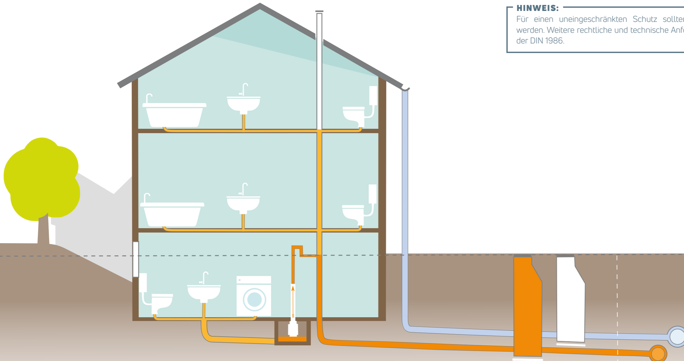
Abbildung 15: Hebeanlage mit Rückstauschleife
