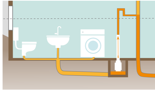
Abbildung 14: Funktionsweise einer Hebeanlage
