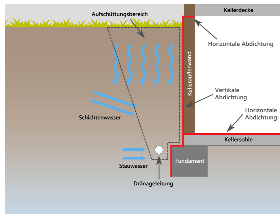
Abbildung 30: Dränageleitung bei nichtstauendem Sickerwasser
