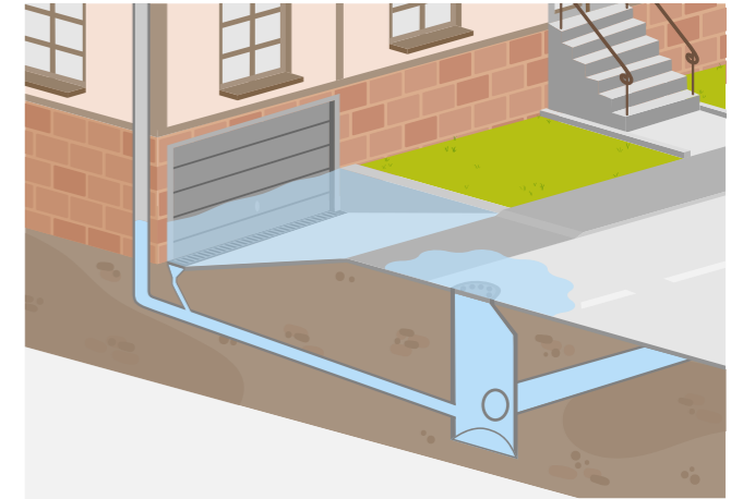
Abbildung 16: Tiefgarage mit Oberflächenabfluss und Rückstau
