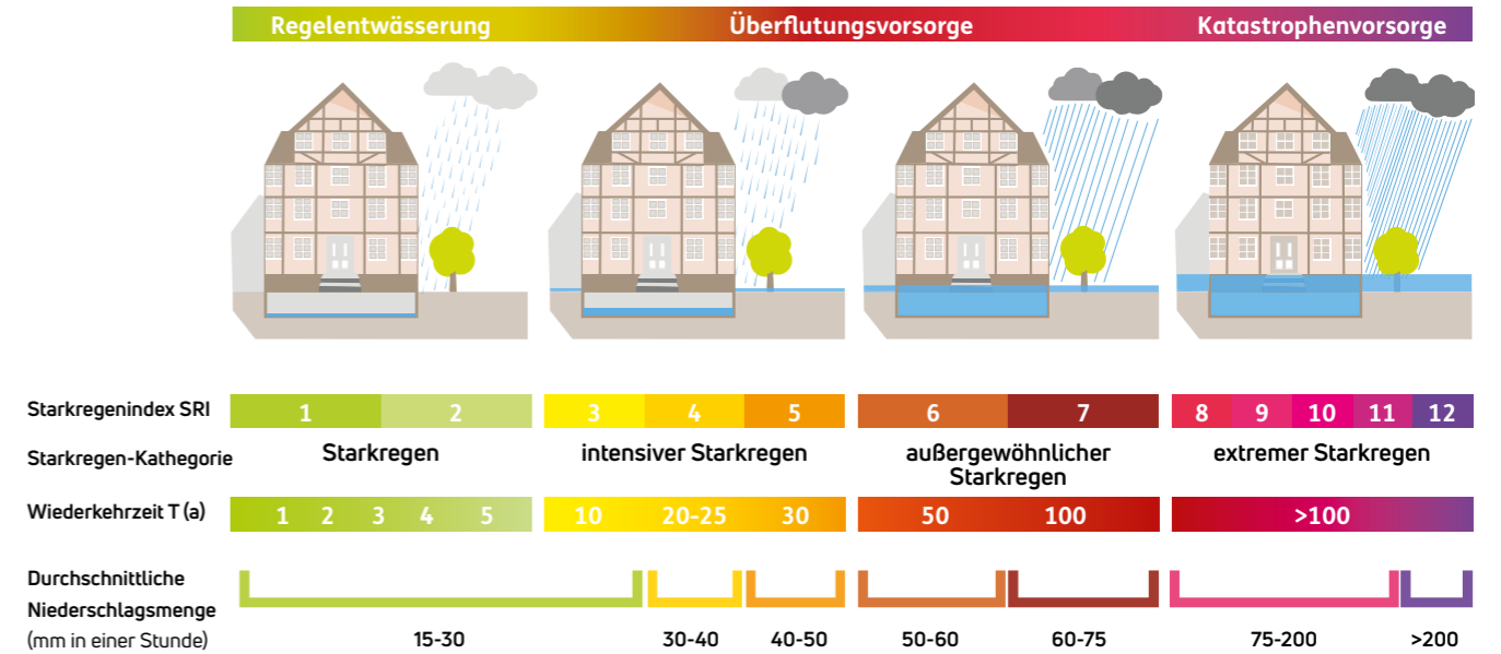
Abbildung 8: Starkregenindex mit Wiederkehrzeiten und Starkregenkategorien. (nach Schmitt et al.)
