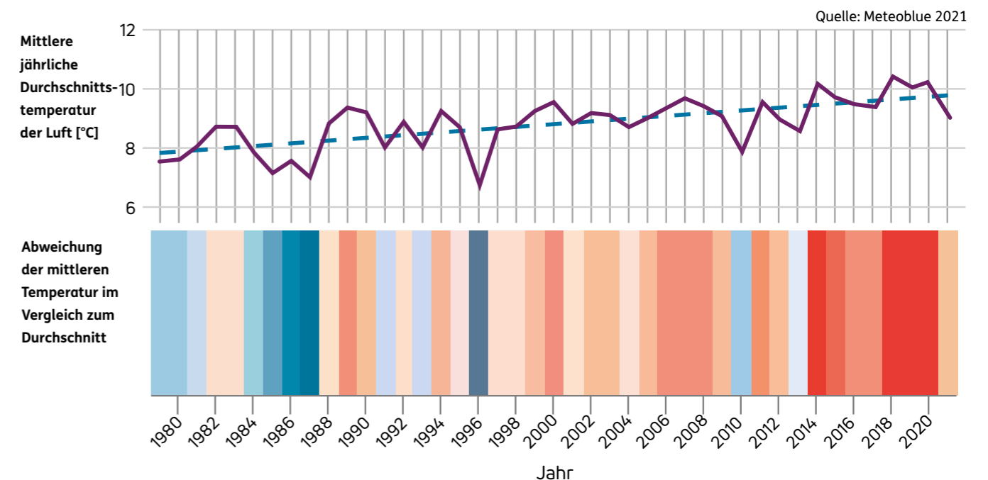
Abbildung 2: Jährliche Mitteltemperatur in Göttingen (lila) mit Trend 1979-2022 (blau-gestrichelt) und jährliche Abweichungen zum Durchschnitt (Temperaturstreifen (blau = kühler als Durchschnitt; rot = wärmer als Durchschnitt)).
