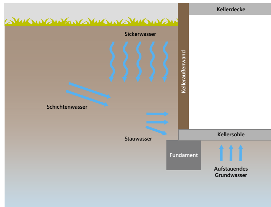
Abbildung 28: Schematische Darstellung von Wasser im Boden
