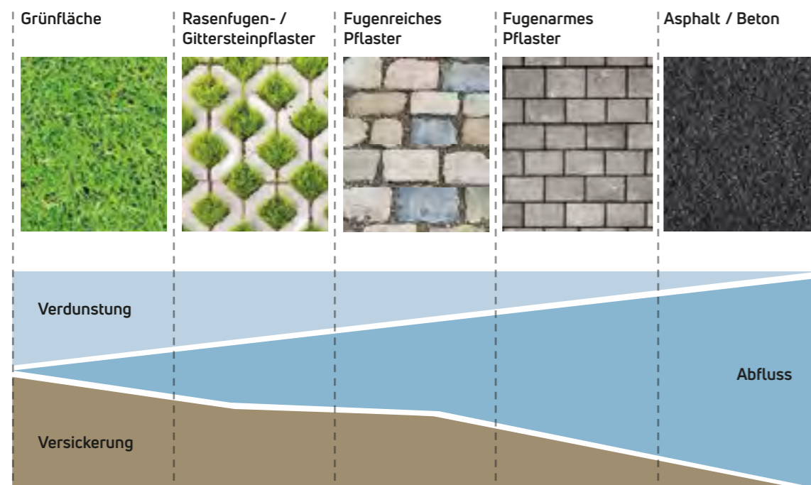
Abbildung 36: Schematische Darstellung der Ausprägung von Abfluss, Versickerung und Verdunstung auf unterschiedlichen Oberflächen (nach Ingenieurbüro Reinhard Beck)
