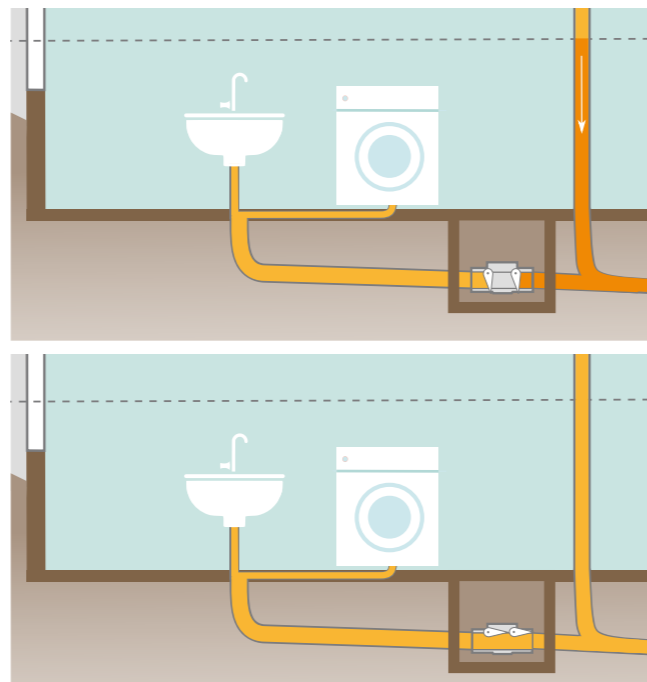
Abbildung 18: Funktionsweise von Rückstauklappen. Oben: Klappe verschließt bei Rückstau die Leitung zum Entwässerungsgegenstand; Unten: ohne Rückstau kann das Abwasser zum Kanalnetz abfließen.
